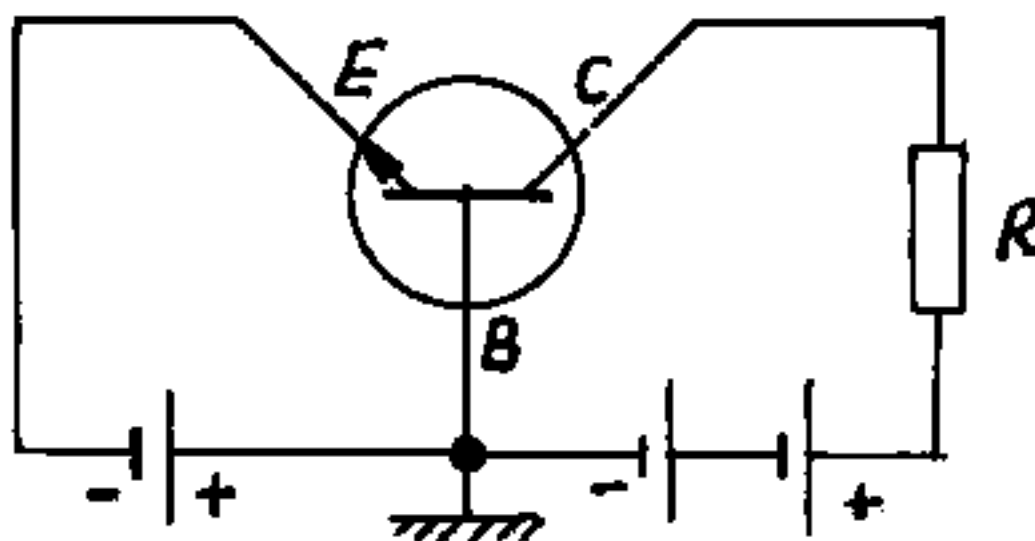
شکل ۱۲: ترانزیستور NPN
