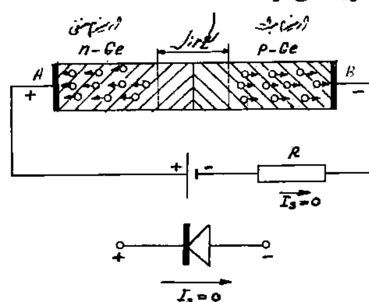
شکل ۹: دیود نیم رسانا در حالت مانع جریان الکتریکی
