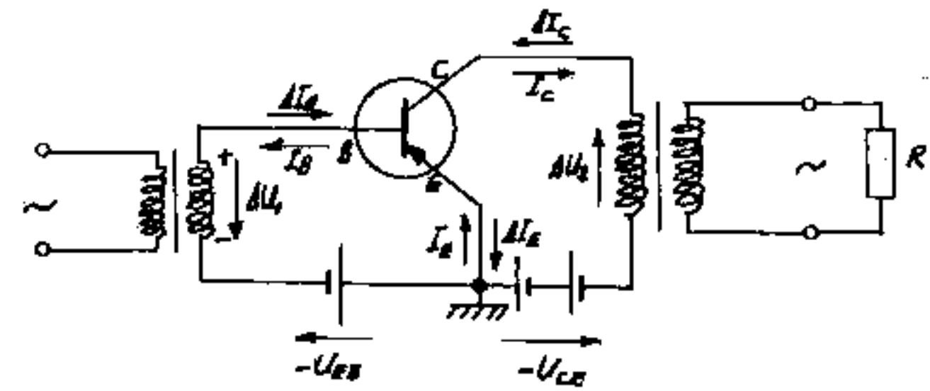
شکل ۱۹ : مدار امی تر
