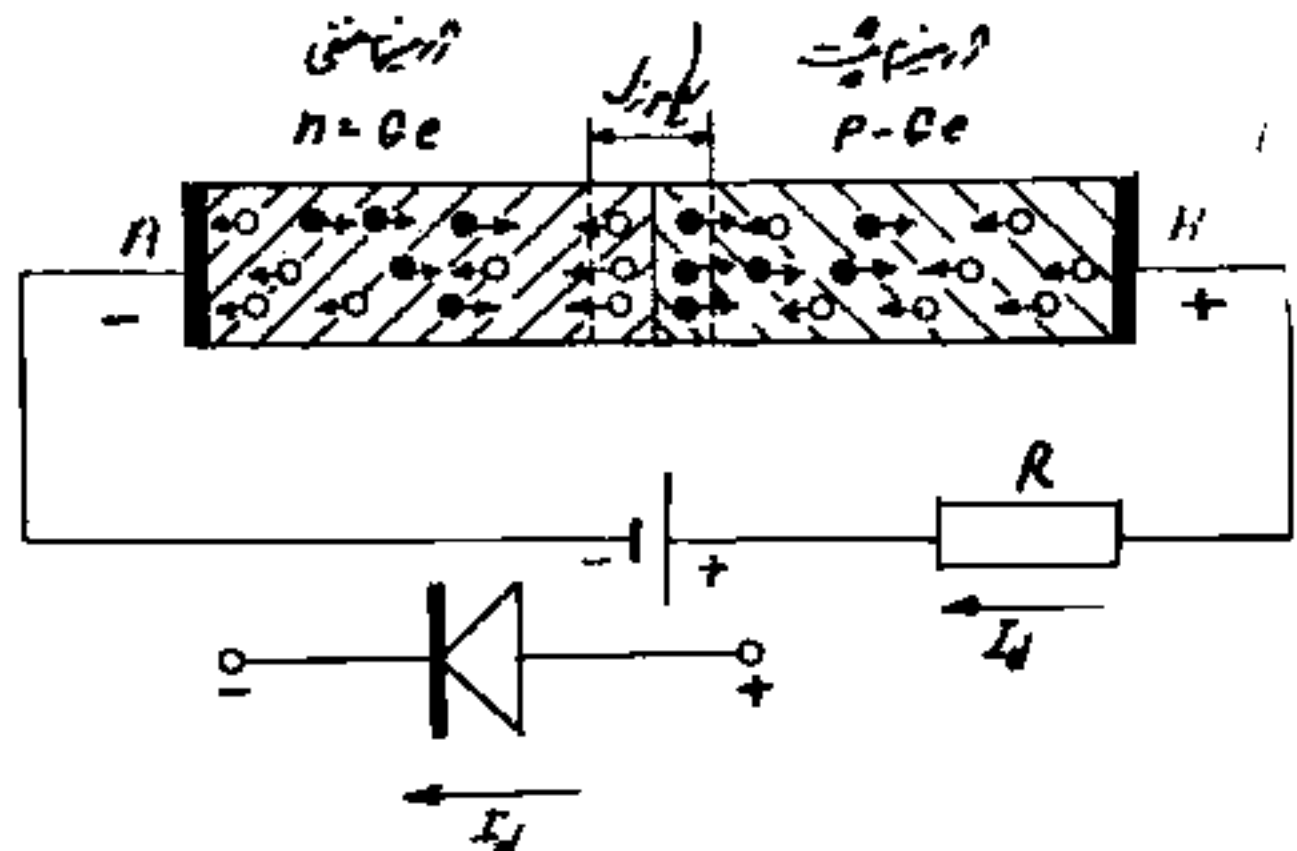
شکل ۱۰: دیود نیم رسانا در حالت عبور جریان الکتریکی
