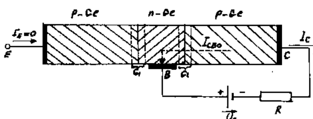
شکل ۱۴: ترانزیستور NPN
