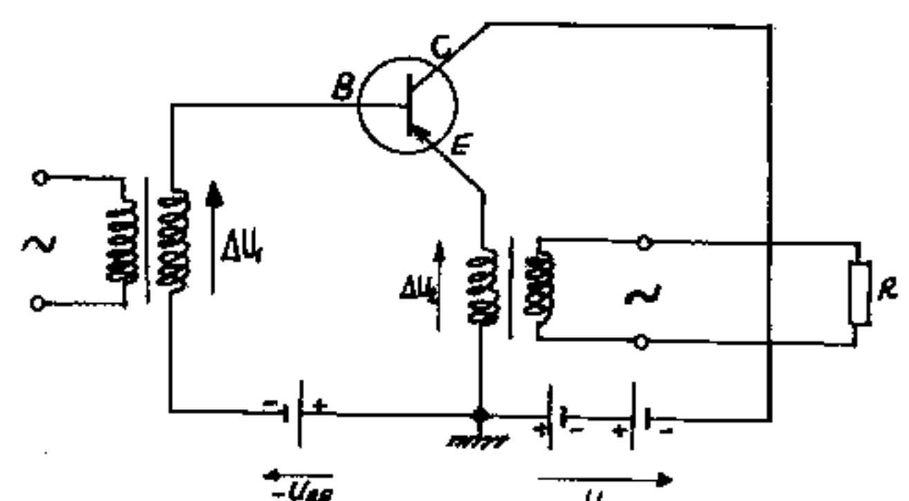
شکل ۲۰ : مدار کولکتور
