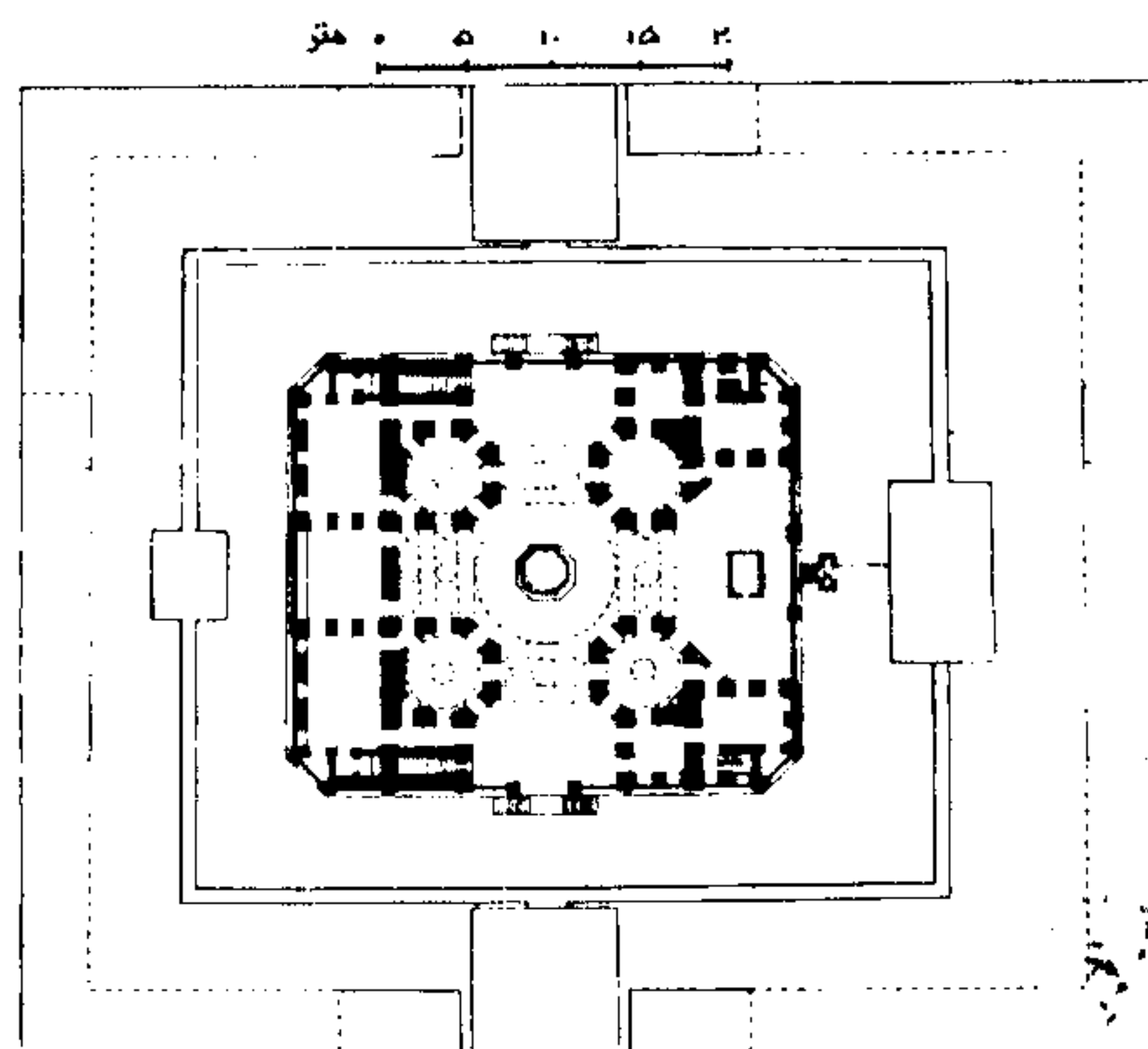
پیش عرضی قصر هشت بهشت اصفهان
