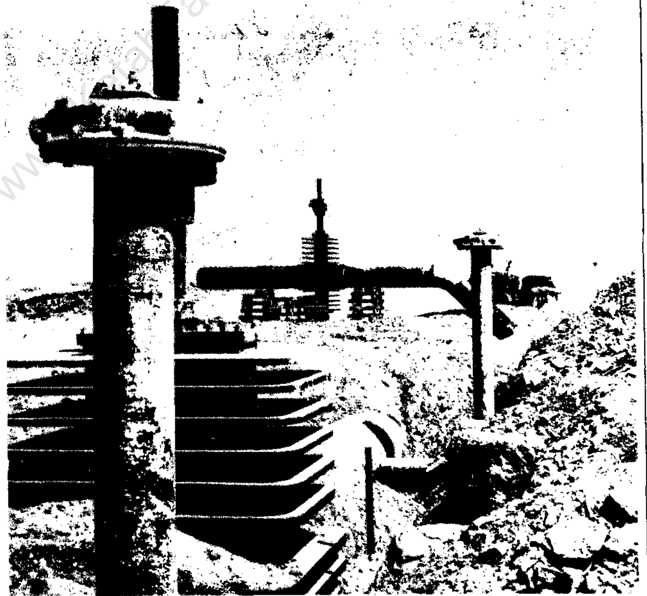
شیر خودکار سی تی ، د کیت والو ، که برای کنترل فشار خط شاه لوله گاز در محل های لازم نصب شده و هرگاه سانچای در خط لوله اتفاق افتد خود بخود جریان گاز را قطع میکند .
